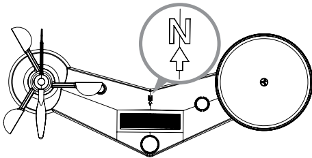
Noordelijke marking bovenop de 7-in-1 sensor.
